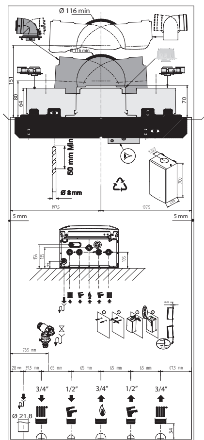
Dima di montaggio
